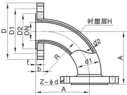
90°弯头
