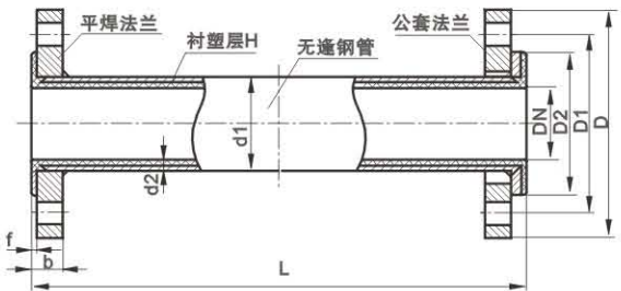
衬里直管
