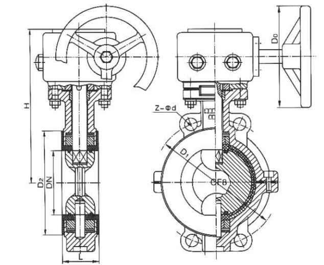
DA371F46/P型对夹式蜗轮传动蝶阀(中线)
