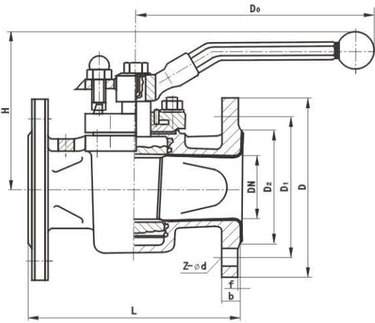
法兰连接旋塞阀 ( 全衬里 , 卡套式 )
