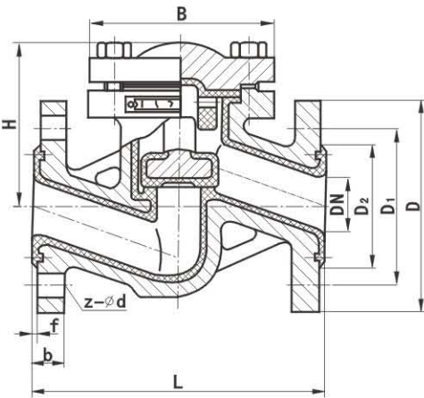
衬氟止回阀标准
