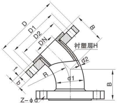
45°弯头
