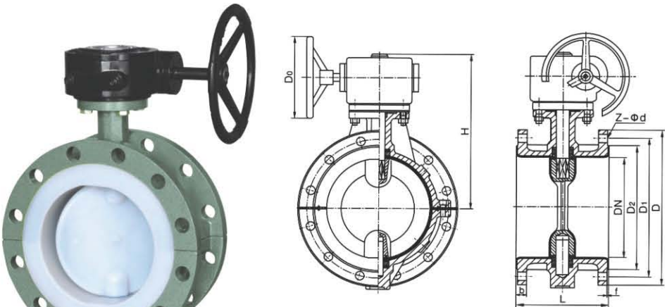
D341F46型法兰连接蜗轮传动蝶阀(中线)
